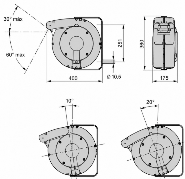
Imagen 4 : Plano devanadera
