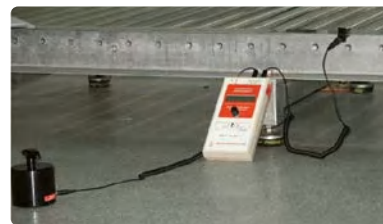
Procedimiento de medición de la resistencia a tierra de un pavimento antielectrostático.
