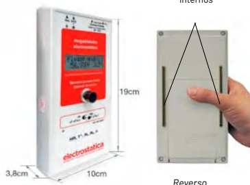
Electrodos internos
